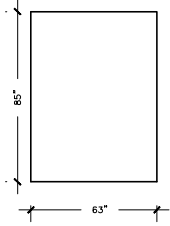
DOUBLE BED W: 63" D: 85" H: 57" SIDE H: 16" PLAT H: 14.5"
