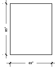
QUEEN BED W: 69" D: 85" H: 57" SIDE H: 16" PLAT H: 14.5"
