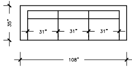
SOFA PLUS W: 108" D: 35" H: 32"
